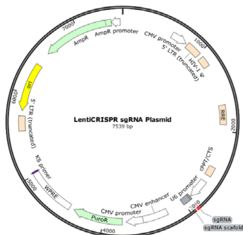
图 3 Edi-HTS™WHG 文库质粒结构
