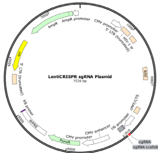
图 3 Edi-HTS™HK 文库质粒结构
