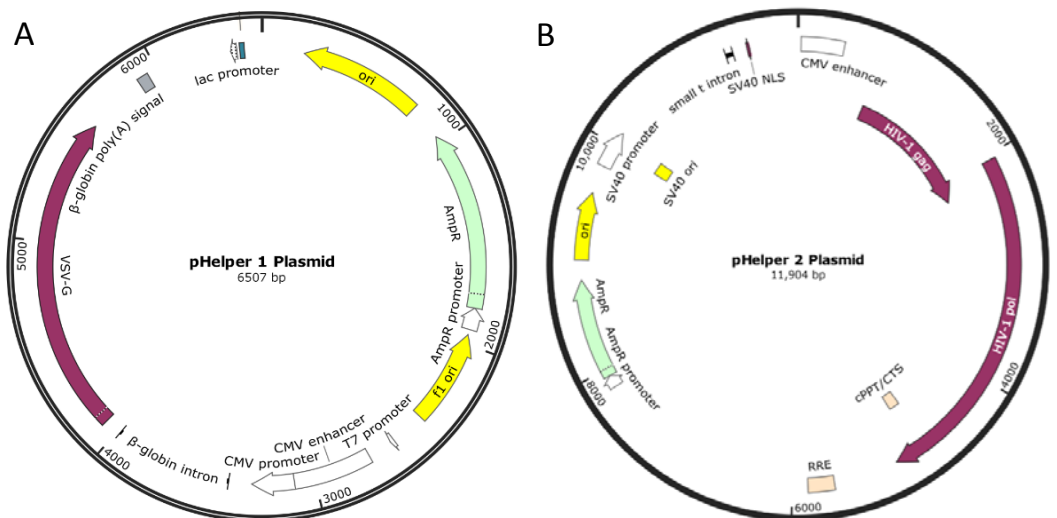
图 4 Edi-HTS™ HP 病毒包装质粒 pHelper 1 和 pHelper 2
