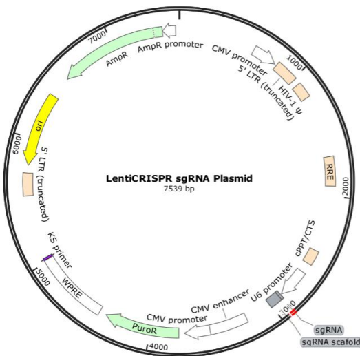
图 3 Edi-HTS™ HKP 文库质粒结构
