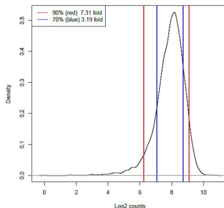
图 1 Edi-HTS™HKP 文库 sgRNA 的分布
