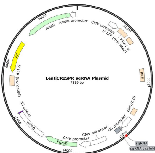
图 3 Edi-HTS™ HTMR 文库质粒结构
