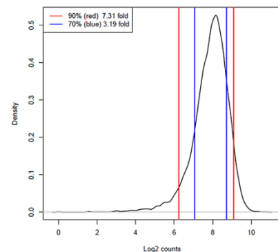
图 1 Edi-HTS™ HT 文库 sgRNA 分布
