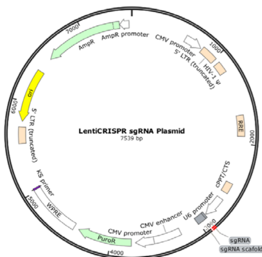
图 3 Edi-HTS™ HT 文库质粒结构
