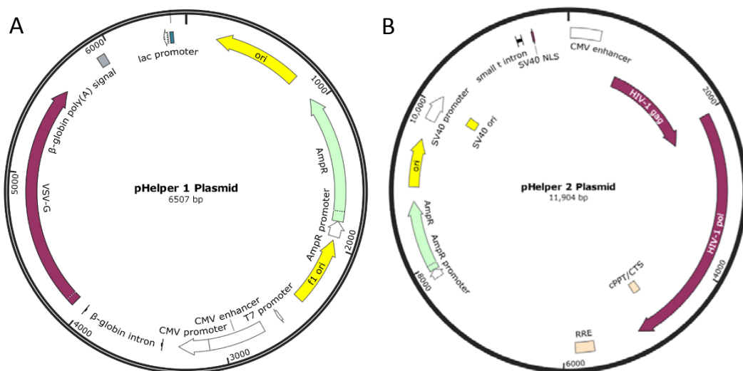
图 4 Edi-HTS™ HT 病毒包装质粒 pHelper 1 和 pHelper 2
